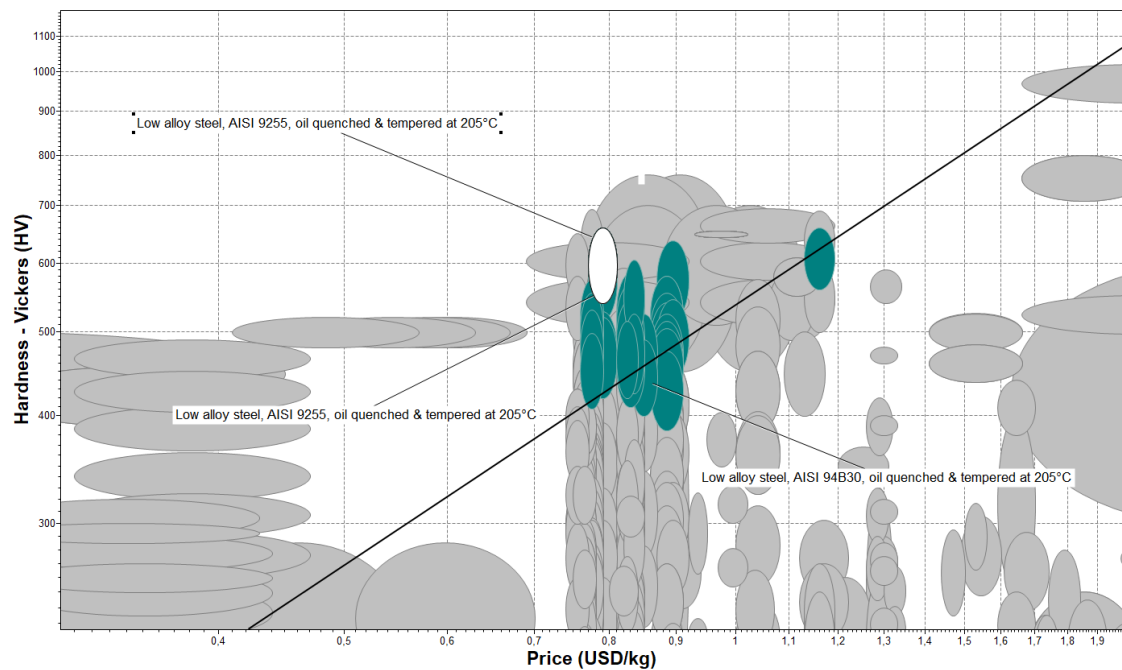
Figura 2: Diagrama de CES Edupack Para acero elegido para los cinceles.
