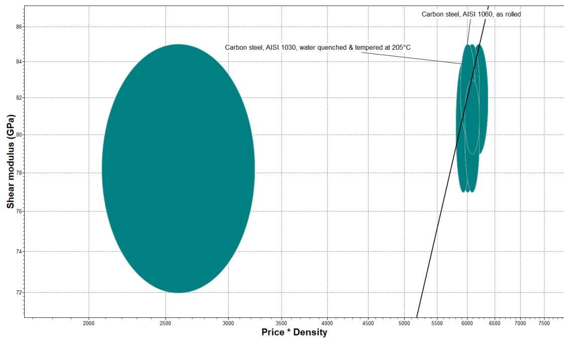
Figura 3: Diagrama de CES Edupack Para bulonería.
